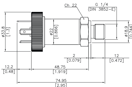
Connector EN 175301-803 Form A
